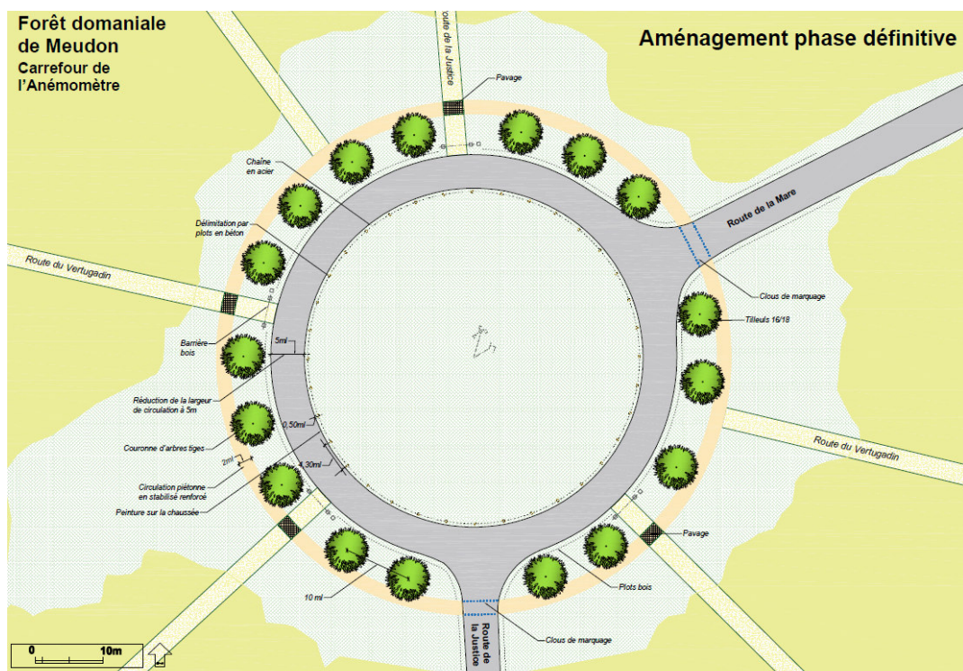
Carrefour de l'anémomètre – Projet (©ONF, S. Meyrier)
